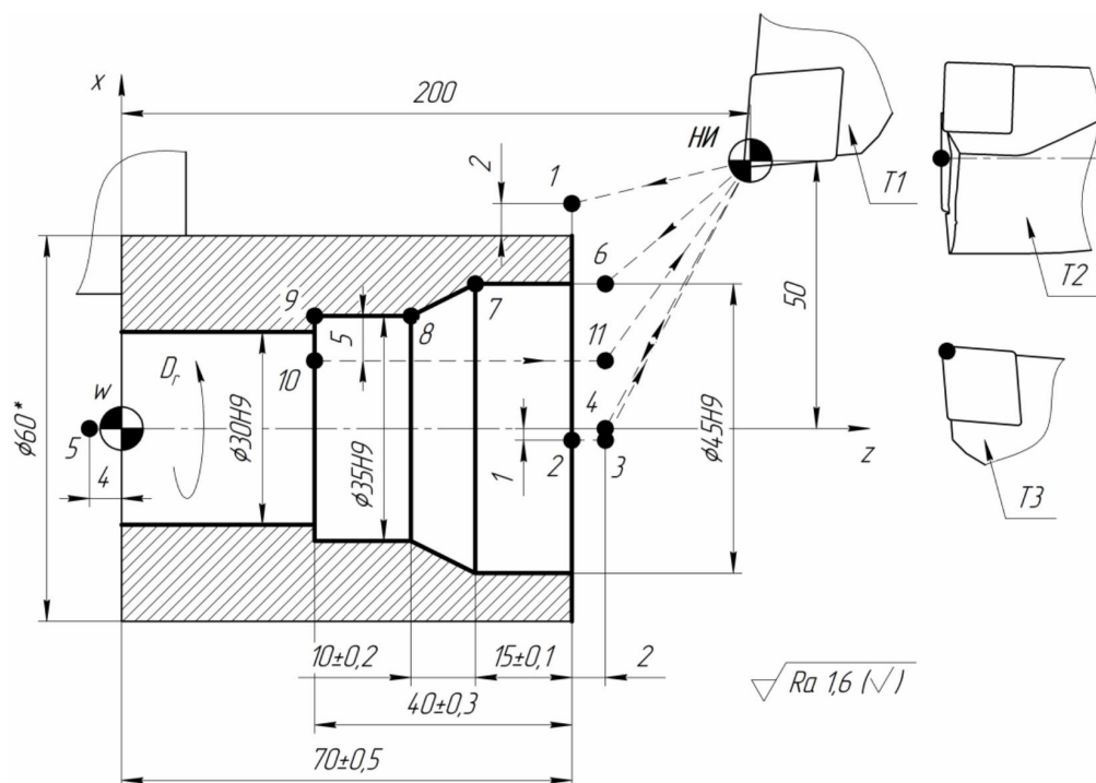
Рисунок 1. Эскиз расчетно-технологической карты
